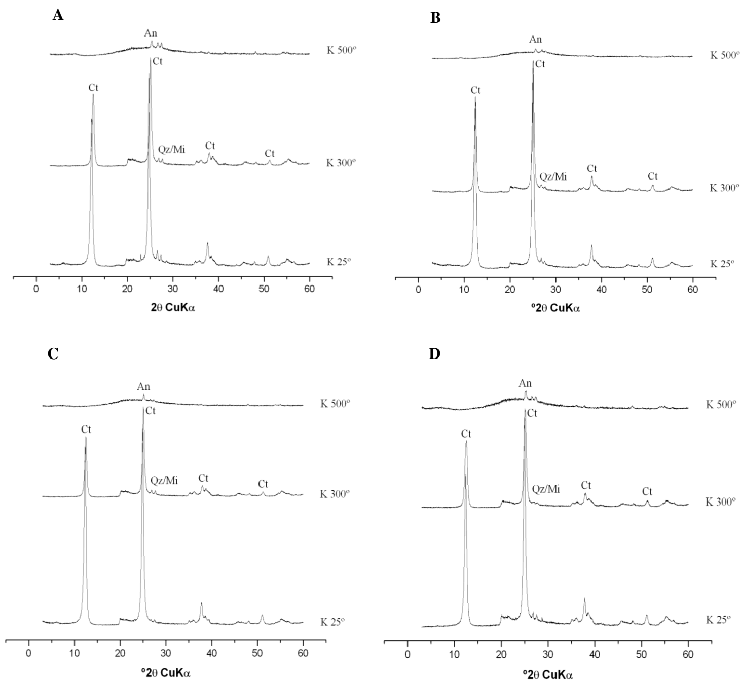
Figura 6. Difratomogramas da fração argila de Argissolo Amarelo com A antrópico: A) 0-20 cm ( Au_1 ) e B) 80-100 cm ( Au_3/Au_4 ); C) Argissolo Amarelo com A moderado: 0-20 cm ( A/AB ) e D) 80-100 cm ( Bt_1 ) da Estação Experimental do Caldeirão (Embrapa/CPAA), Irlanduba – AM.
