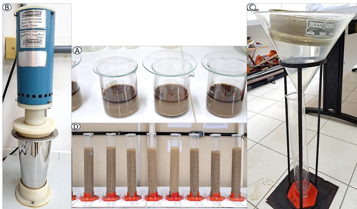
Figura 24 — Procedimentos da análise granulométrica (A. amostra em processo de decantação; B. amostra no agitador magnético; C. amostra sendo lavada com água destilada; D. Amostra de finos decantando para a pipetagem).
