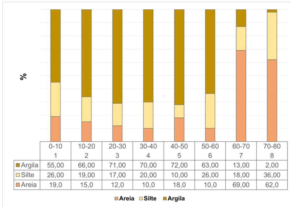
Figura 53 — Análise granulométrica do perfil 1, falésia 1.
