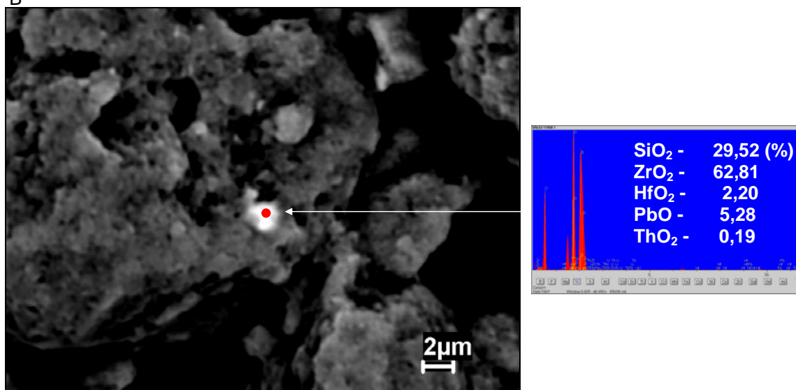
FIGURA 7.30 – Imagens da MEV da amostra SR-L-53 com seus respectivos EDS.
