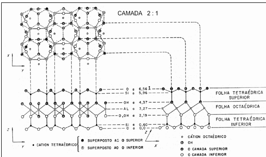
FIGURA 2.4 – Projeções sobre [001], [100] e [010] da camada 2:1 (Baseado em LUCAS, 1962, e compilado de ALVES, 1990).
