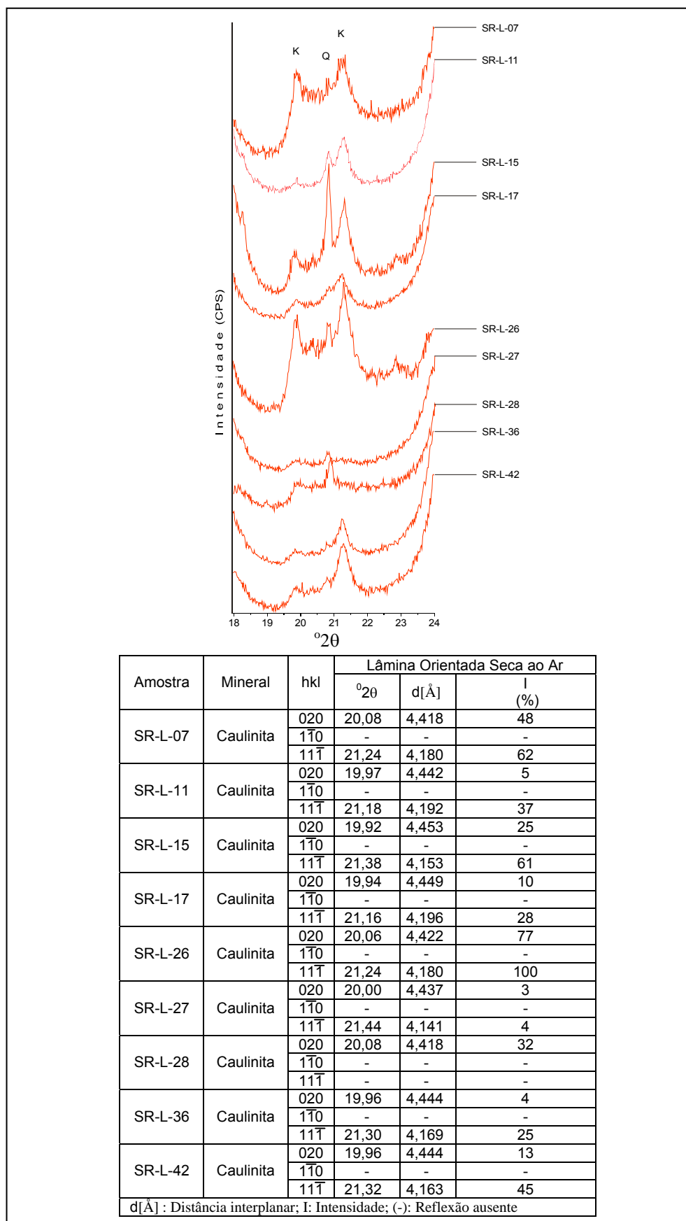
FIGURA 7.4 – Difractogramas de 9 amostras da Fazenda Santa Cecília mostrando o comportamento das reflexões da caulinita na faixa onde é determinado o índice de Hinckley. K - caulinita; Q - quartzo
