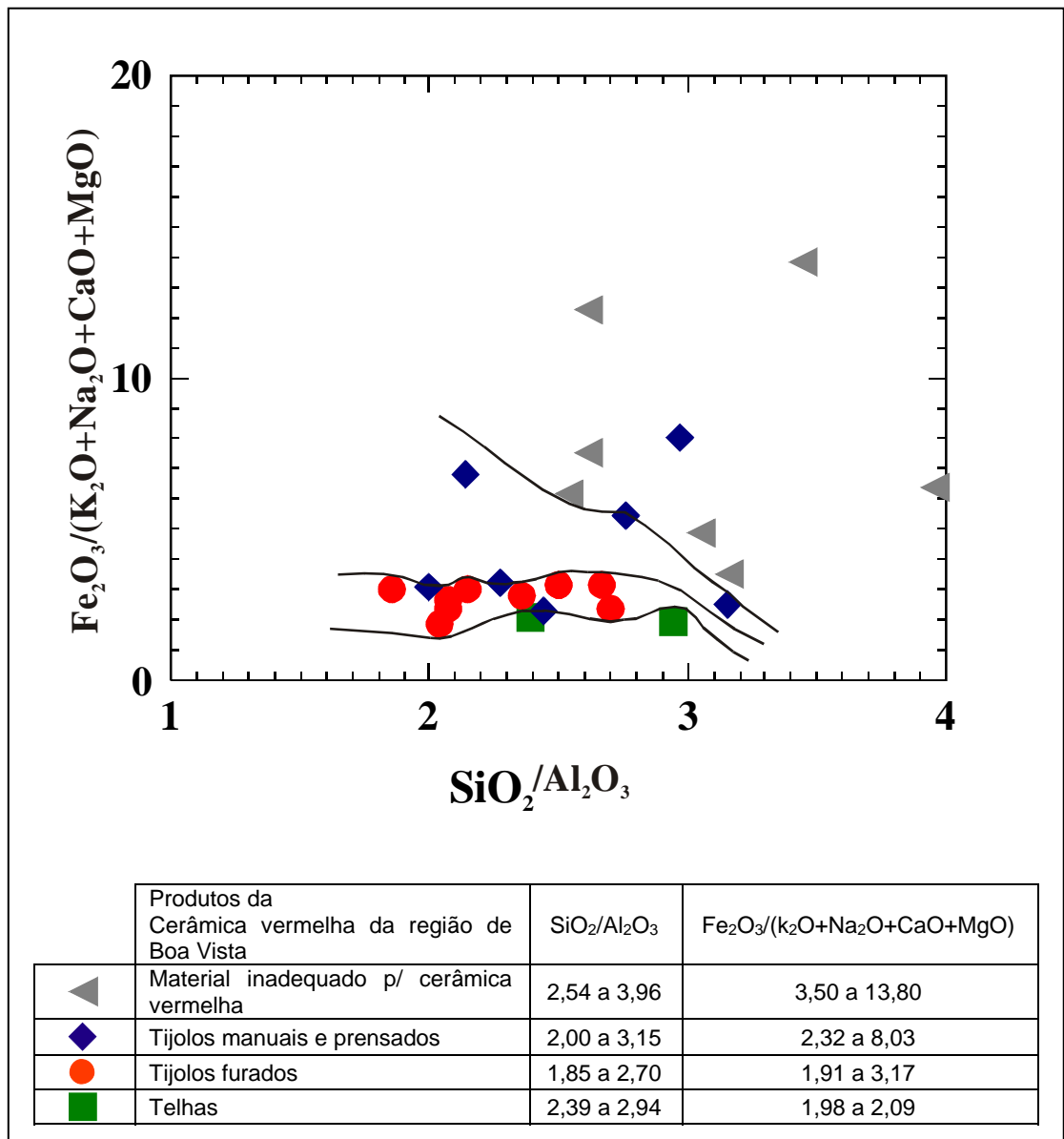
FIGURA 9.2 – Quimismo versus produtos da cerâmica vermelha obtidos nos testes específicos para tijolos e telhas nos sedimentos argilosos da região de Boa Vista
