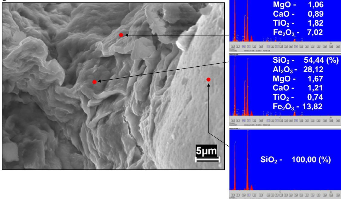
FIGURA 7.49 – Imagens de MEV da amostra SR-L-22 com os seus respectivos EDS, onde as esmectitas apresentam texturas crenuladas
