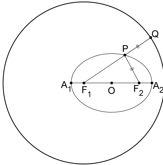
Figura 3.6: elipse: circunferência diretora
