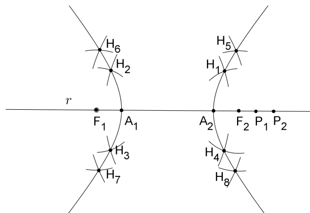
Figura 3.11: hipérbole: construção
