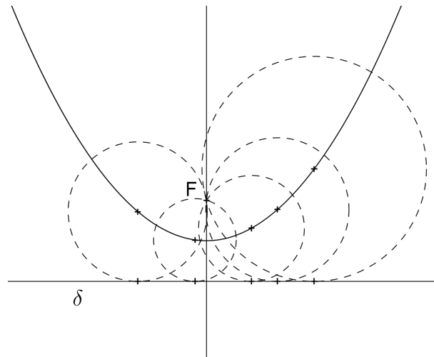
Figura 3.18: parábola: construção
