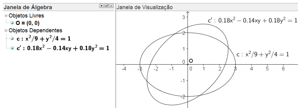
Figura 5.9: Rotação da elipse
