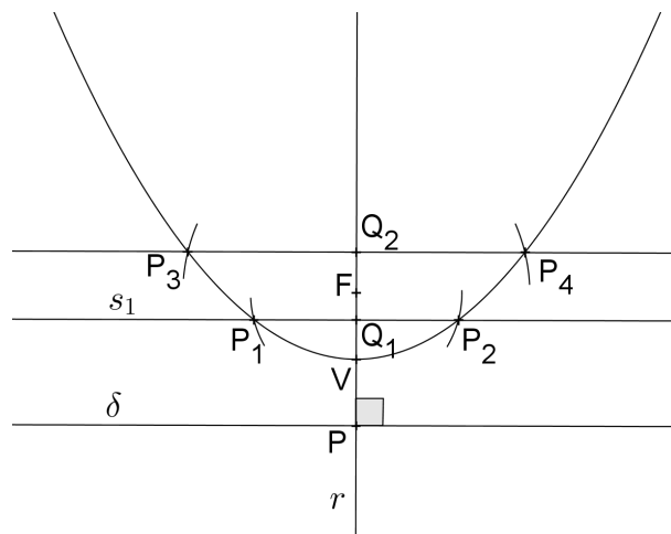
Figura 3.17: parábola: construção
