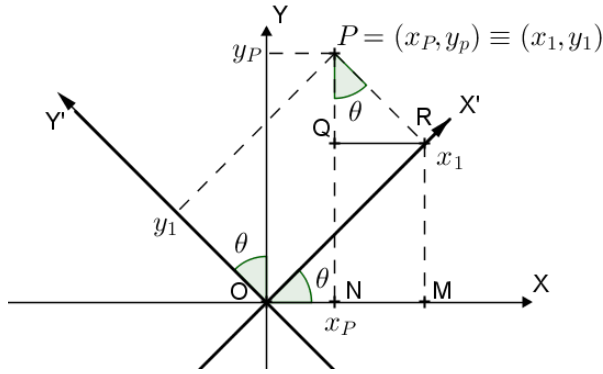
Figura 4.7: Rotação
