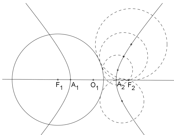
Figura 3.14: hipérbole: circunferência diretora
