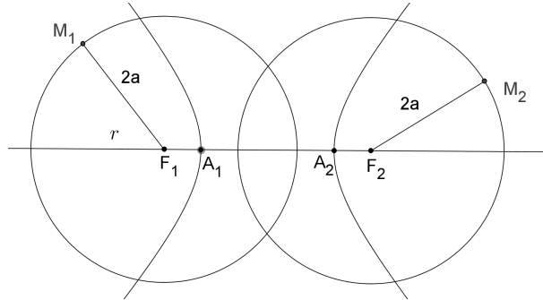
Figura 3.12: hipérbole: circunferência diretora
