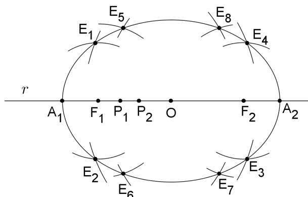
Figura 3.4: elipse: construção
