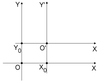
Figura 4.1: Translação
