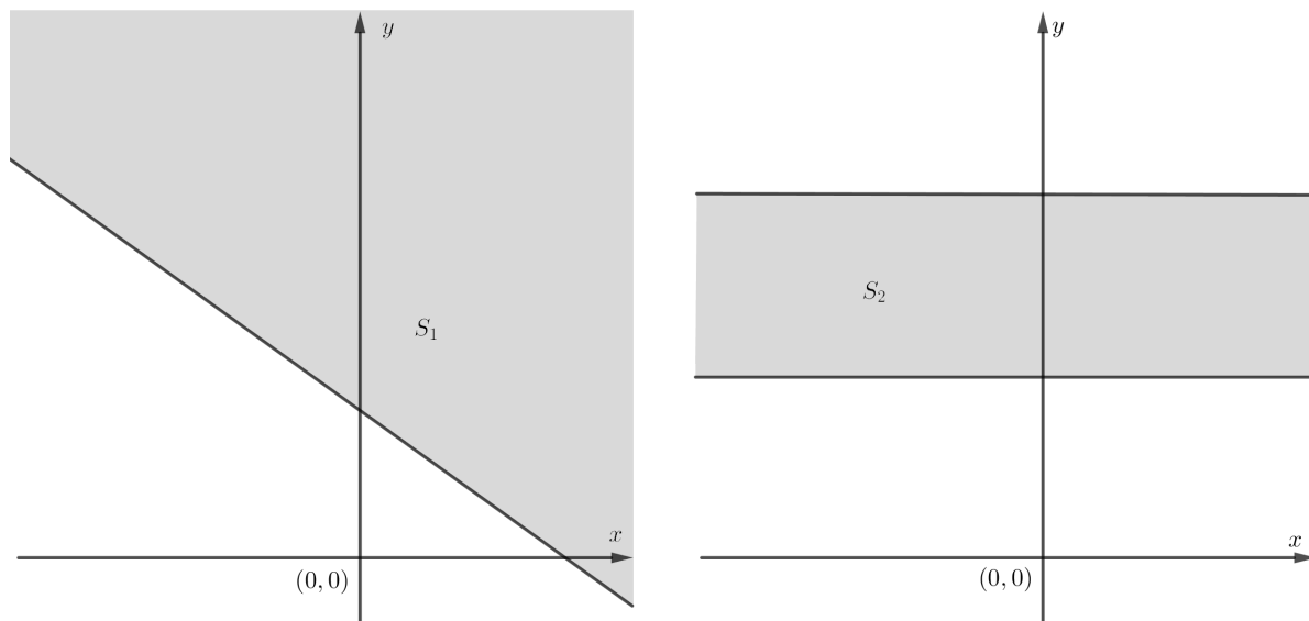
Figura 3.5: Região ilimitada sem vértices
