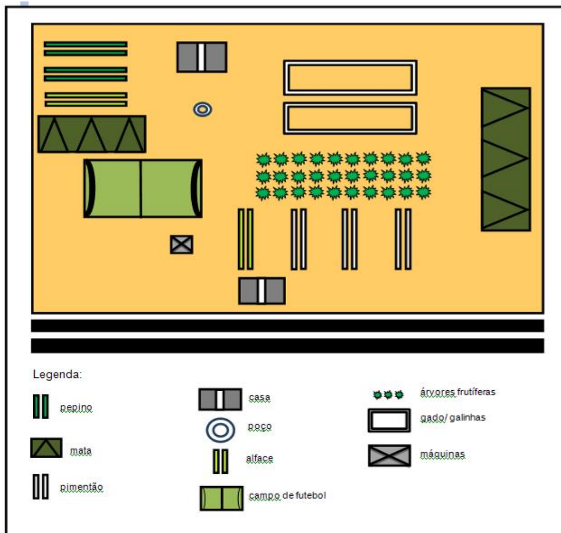
Figura 17 ã Croqui de unidade de produção na Rua Carlos Braga, Iranduba/AM
