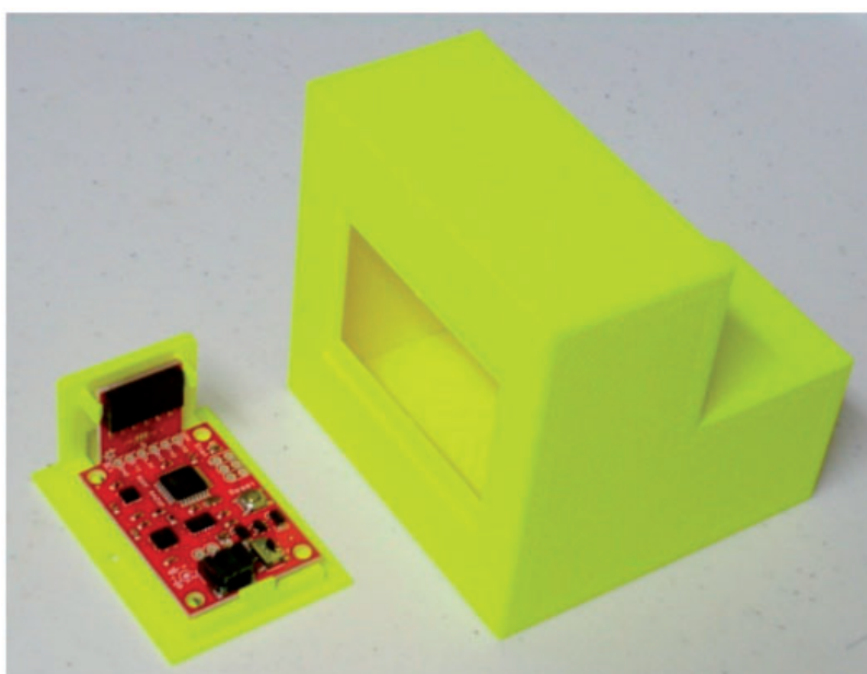
Figura 3.3: Manipulativo Físico com placa e sensores. Fonte: Ha e Fang (2018)
