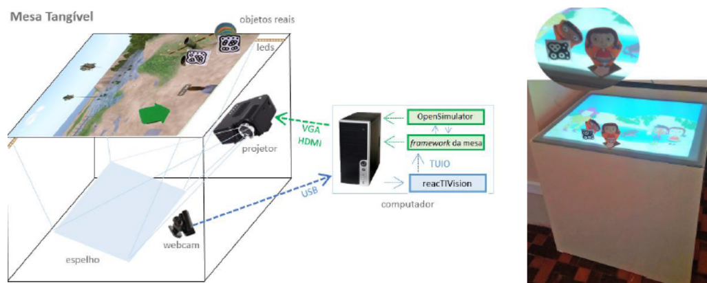
Figura 3.16: Estrutura e componentes da mesa tangível.
