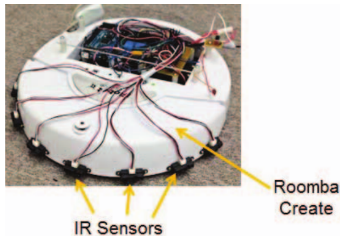
Figura 3.5: RoCr com Arduino e sensores infravermelho integrados. Fonte: Azad e Hashemian (2016)
