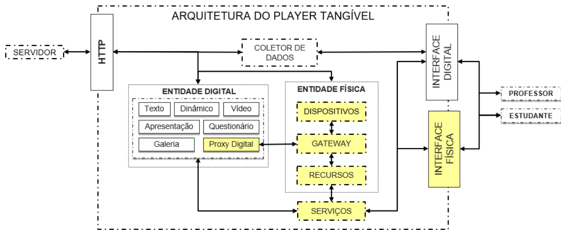
Figura 4.9: Arquitetura do Player Tangível
