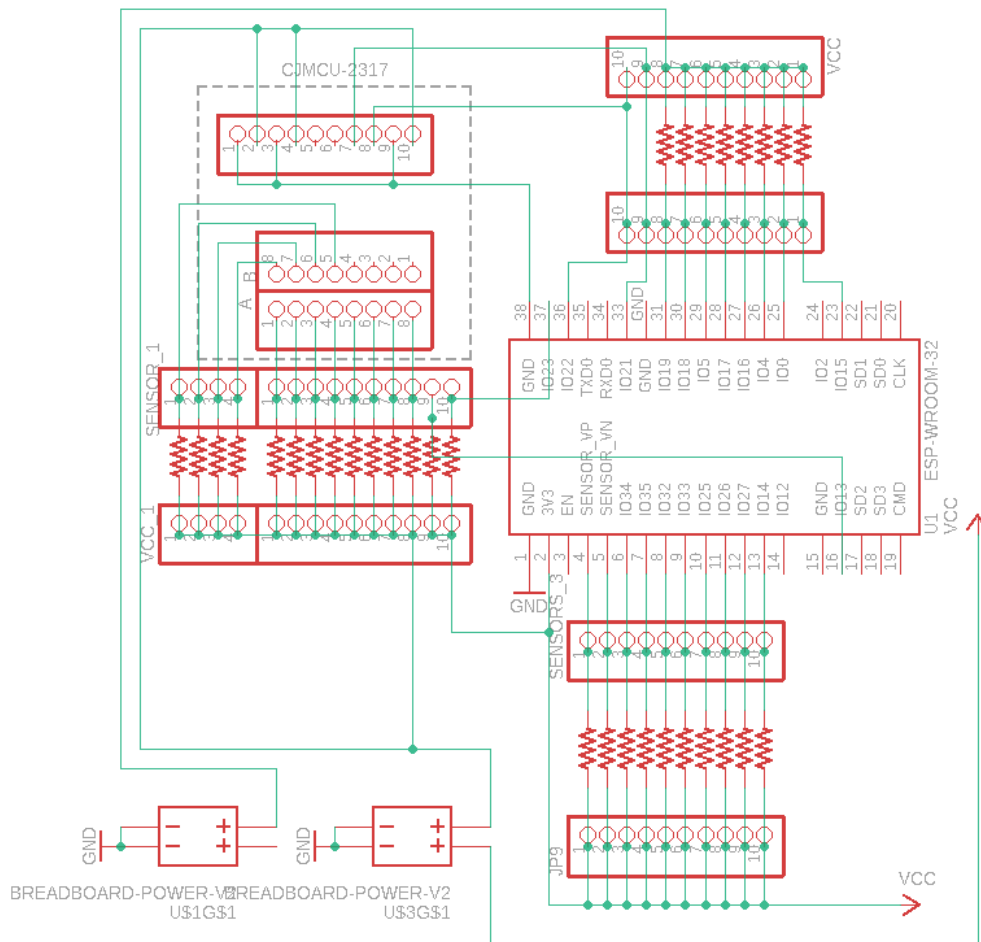
Figura 4.27: Esquemático do Circuito Elétrico utilizado no Player Tangível
