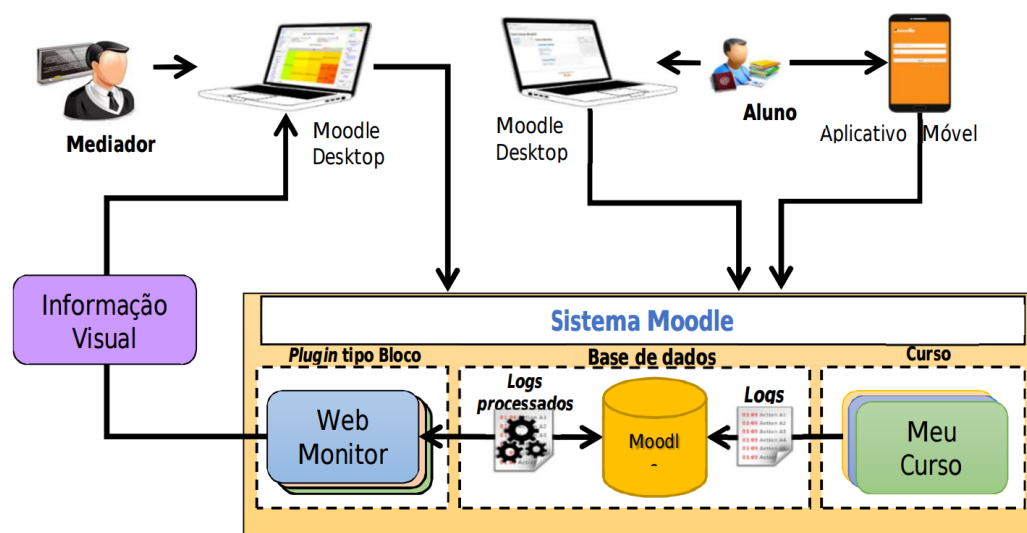
Figura 3.20: Arquitetura do WebMonitor. Fonte: Lucena et al. (2015)
